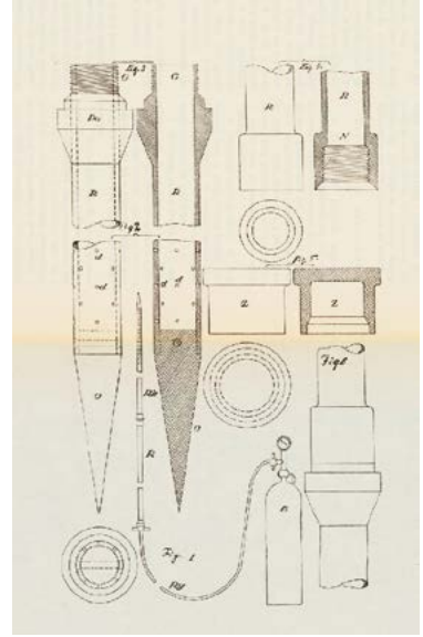
Przewoźne urządzenie gaśnicze na dwutlenek węgla projektu Józefa Tuliszkowskiego
