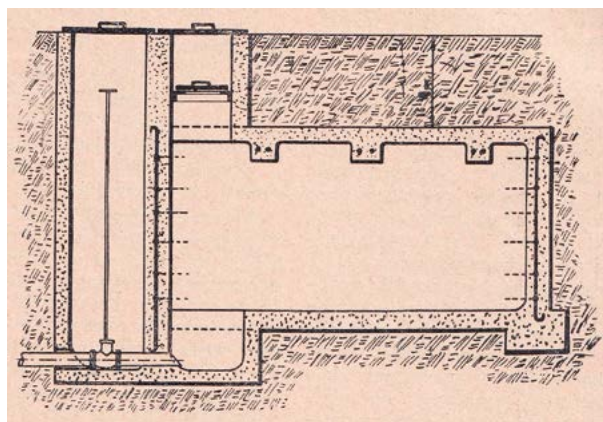
Zbiorniki na wodę projektu Tuliszowskiego
