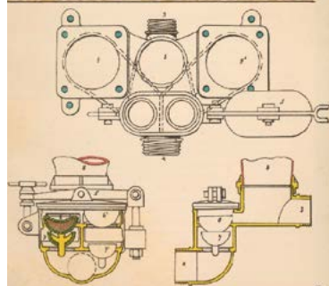
Przekrój sikawki
