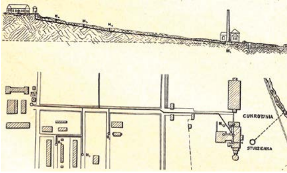
Wieża ciśnień i wodociąg projektu Tuliszkowskiego
